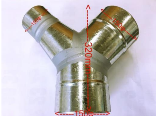
【従来のブリキ製のY字管】
