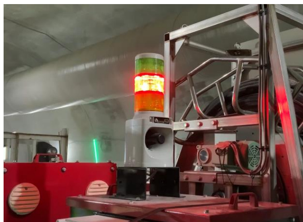
写真8 異常発生時警報装置(音声連動)
