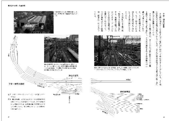
配線の構造を図でわかりやすく解説
