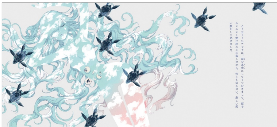
『瓶詰地獄』
