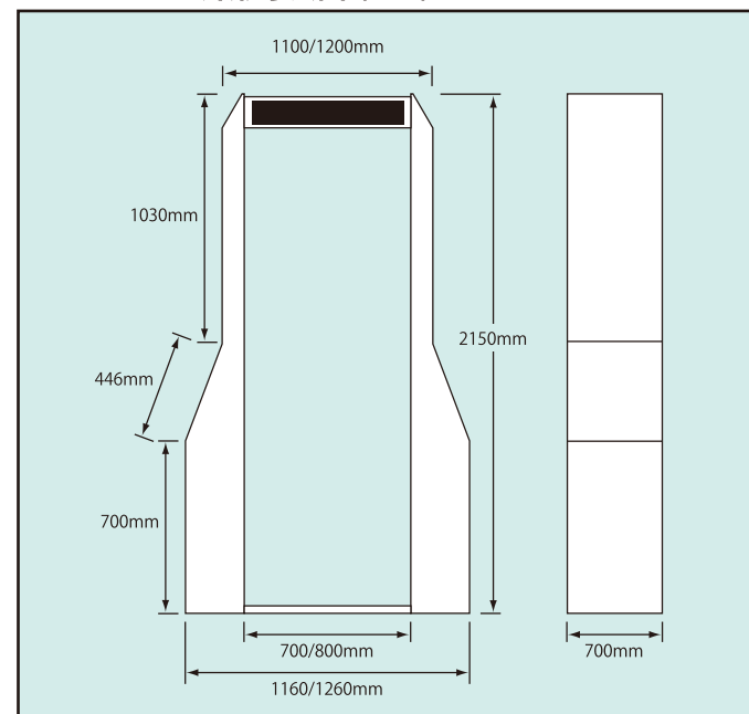
CSG-100/200 外形寸法図 (mm)
