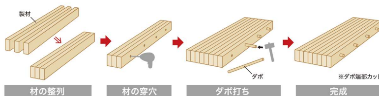
BSボードの製造プロセス
