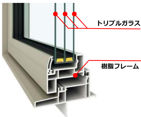
「APW430」製品断面図
