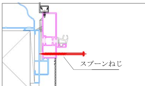
②スプーンネジ取付け断面図
