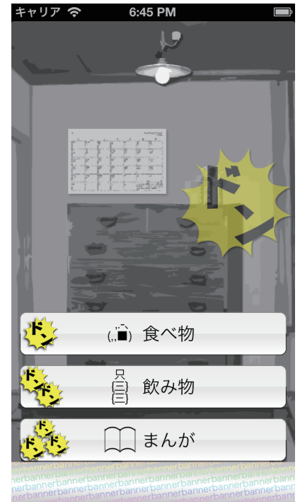
ゲーム画面
