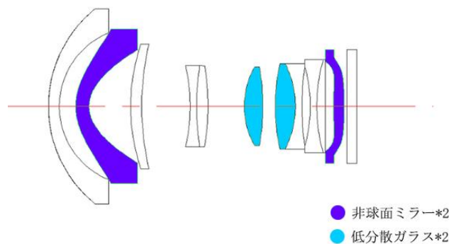
レンズ構成図
