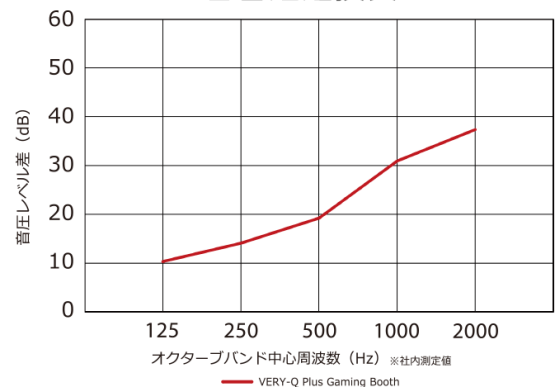
音響透過損失
