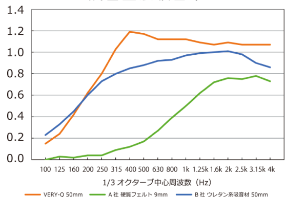
残響室法吸音率
