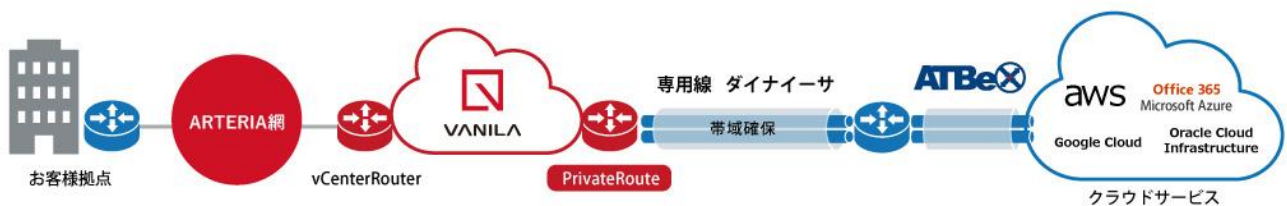
「VANILA PrivateRoute (CloudConnect Dedicated タイプ)」ATBeX 接続 提供イメージ
