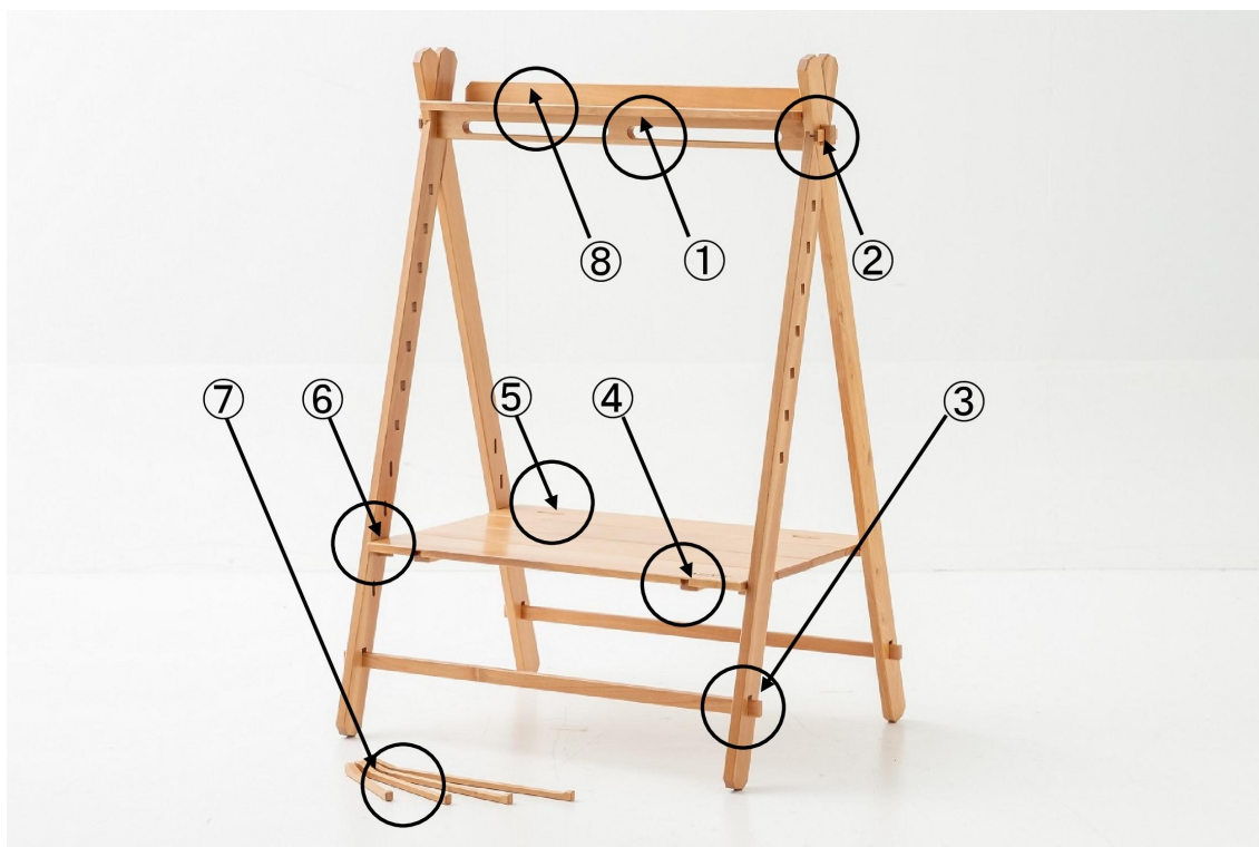
8つの接合技
