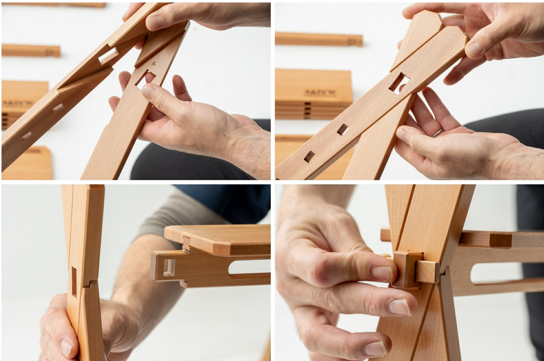
アイカキ接合とクサビ接合
