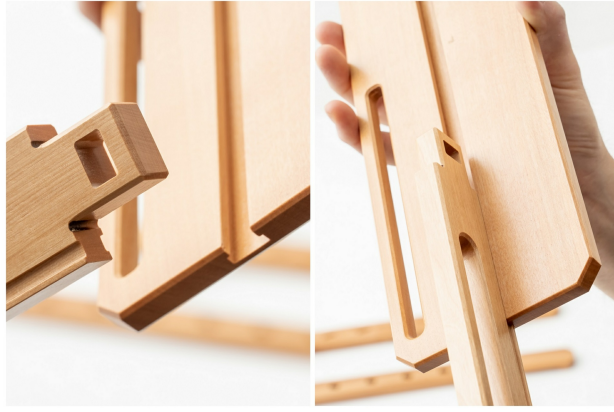
T溝接合
