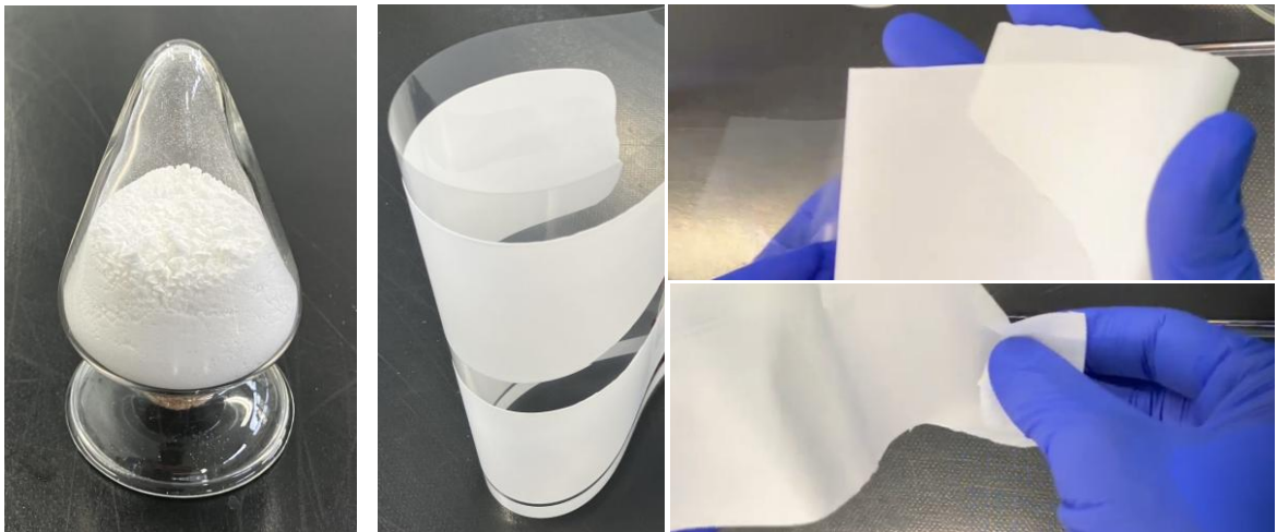
水系複合準固体電解質(3D-SLISE)(左)、3D-SLISE を塗布・乾燥し、作成したシート(右)
