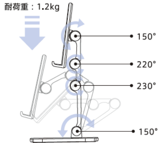
耐荷重：1.2kg ヒンジ可動範囲
