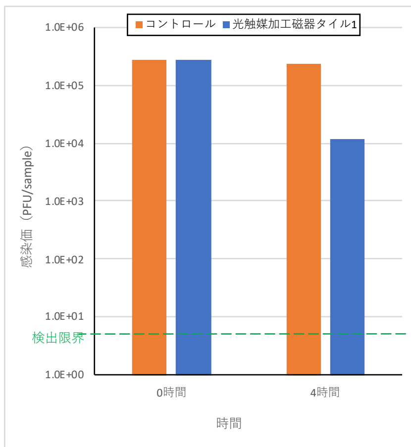
図 1. 光触媒加工磁器タイル 1 によるウイルス感染価の推移
