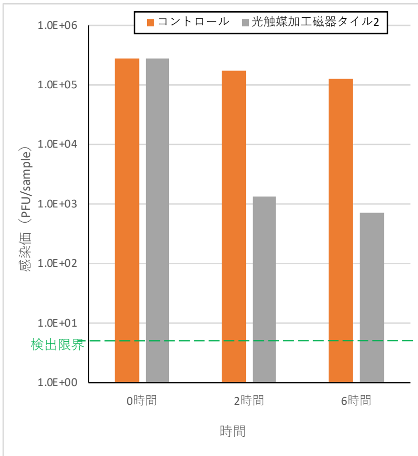
図2. 光触媒加工磁器タイル2によるウイルス感染価の推移
