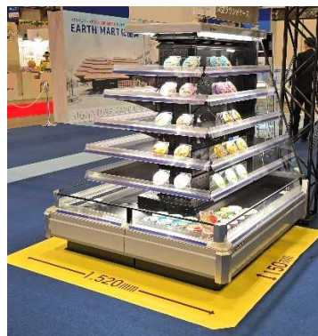
別置型セミ多段オープンショーケース
