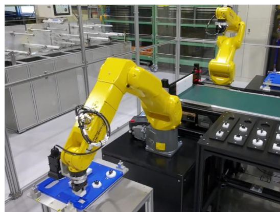
産業用ロボットと搬送用ロボット組み合わせた研修機材
