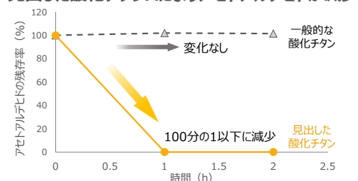
図2. 見出した酸化チタンAによるアセトアルデヒド分解 酸化チタンを含む液をシャーレに塗り、アセトアルデヒドガスを約100ppm注入・密閉し、1.0 mW/cm 2 の紫外線を照射したあと、濃度の時間変化を調べた。
