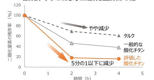
図3. 酸化チタンによる二酸化窒素分解 酸化チタンを含む液をシャーレに塗り、二酸化窒素ガスを120ppm注入・密閉し濃度の時間変化を調べた。
