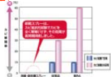
カビ抵抗性試験結果(出光77菌法による)
