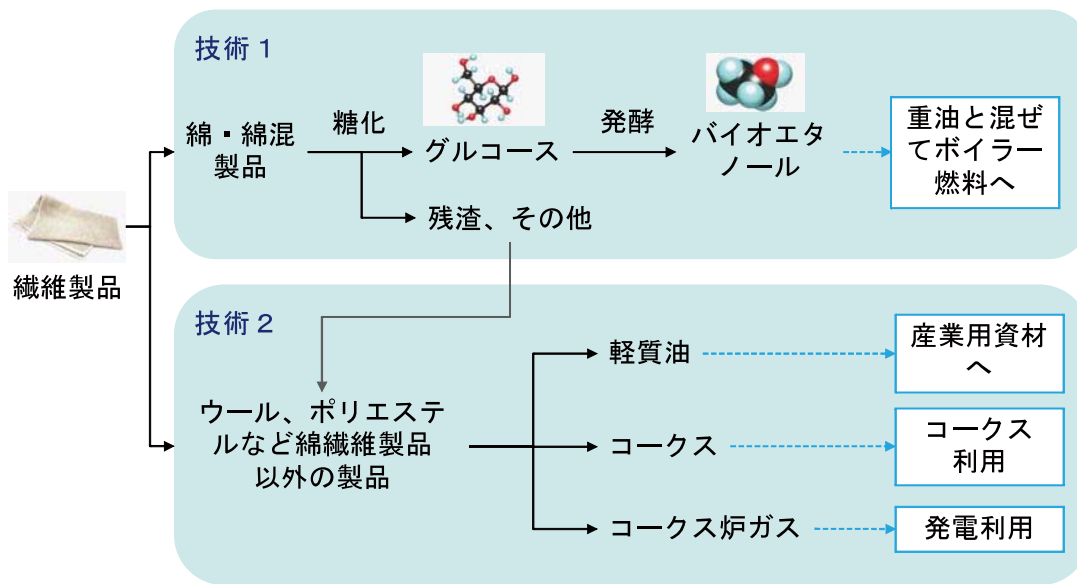
図2.FUKU-FUKU プロジェクトのリサイクル技術
