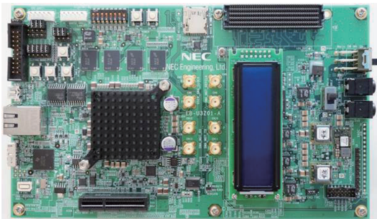
USB3.0開発キット X マザーボード
