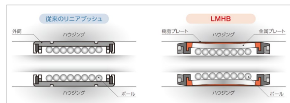
従来のリニアブッシュと「LMHB形」の構造比較
