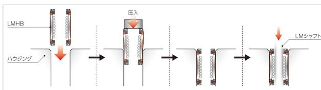
圧入によるハウジングへの組付け方法
