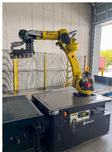
RockyOne 本体
