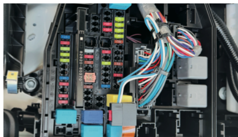
Secure FUSE 取付時イメージ（ランドクルーザー300用）
