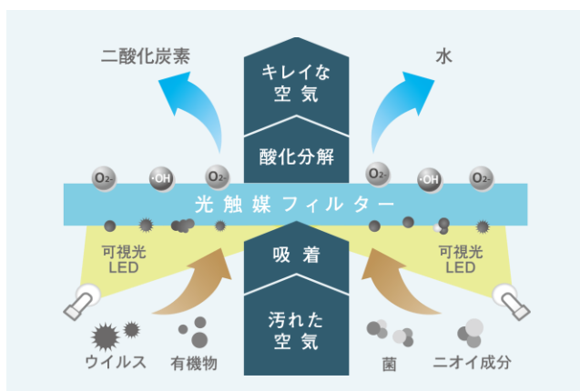
<光触媒のメカニズム>
