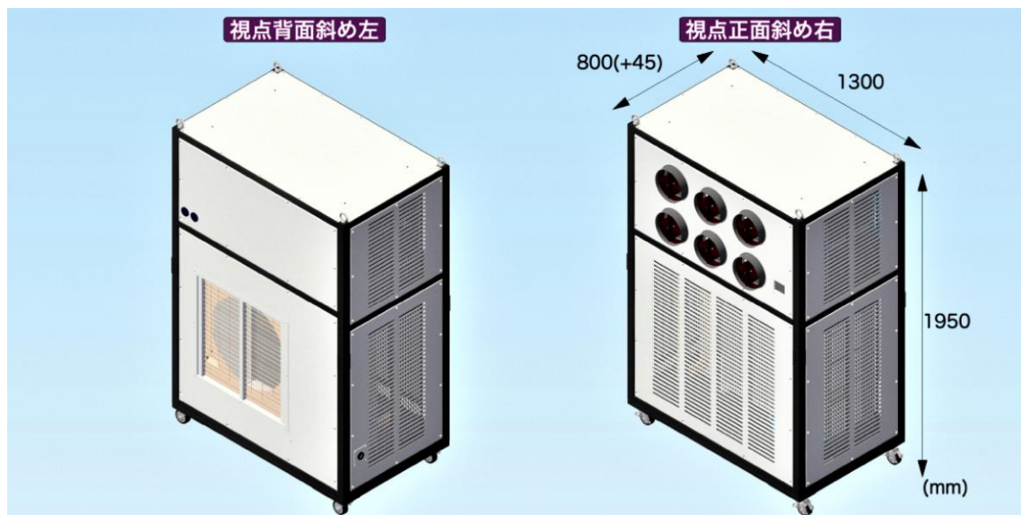
<可搬式空調機>
