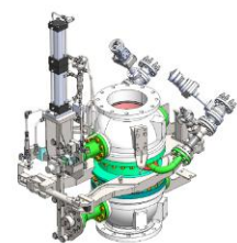
図2：アンモニア用緊急離脱システム（ERS）イメージ
