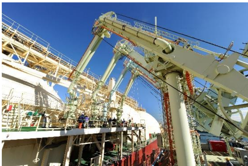
TBG 製 ローディングアーム
